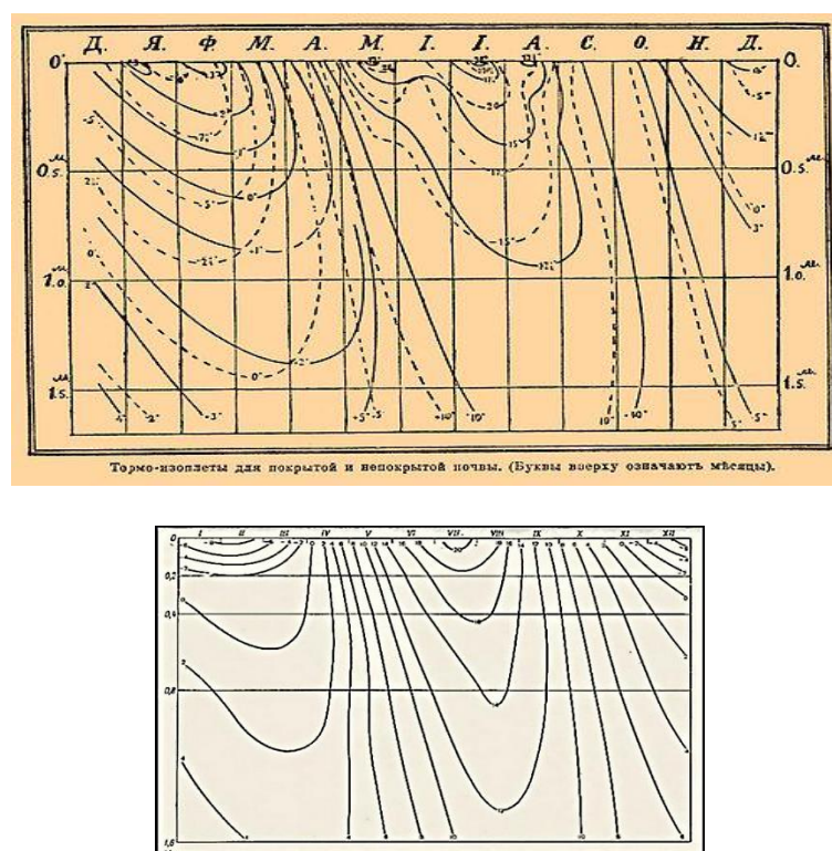
Рисунок – Изоплеты температуры почвы для Санкт-Петербурга.
